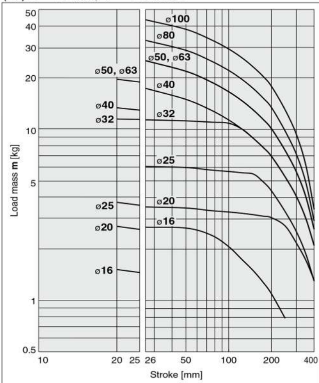
(17) L = 50 mm, V = 400 mm/s
